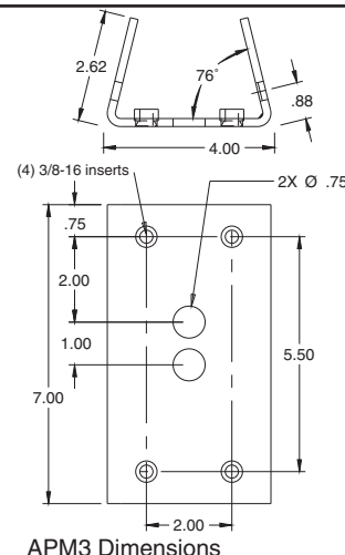
APM3 Dimensions
